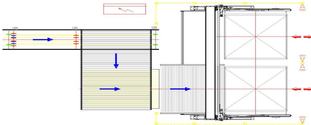
SIRLAMA BANDI ÇIKIŞI VE FIRIN GİRİŞİ STOK SİSTEMLERİ / GLAZING LINE EXIT AND KILN ENTRANCE STORAGE
